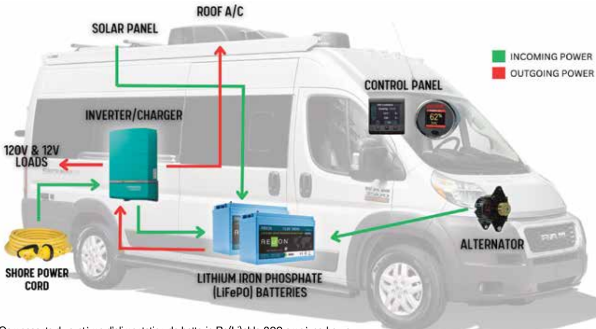
Composants du système d'alimentation de batterie Re(Li)able 200 ampères-heure
