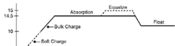
Profil de charge
