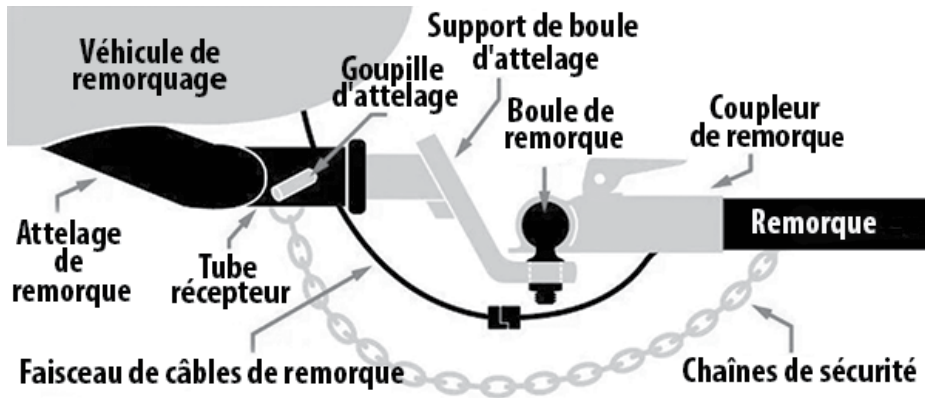
Composants de remorquage typiques
