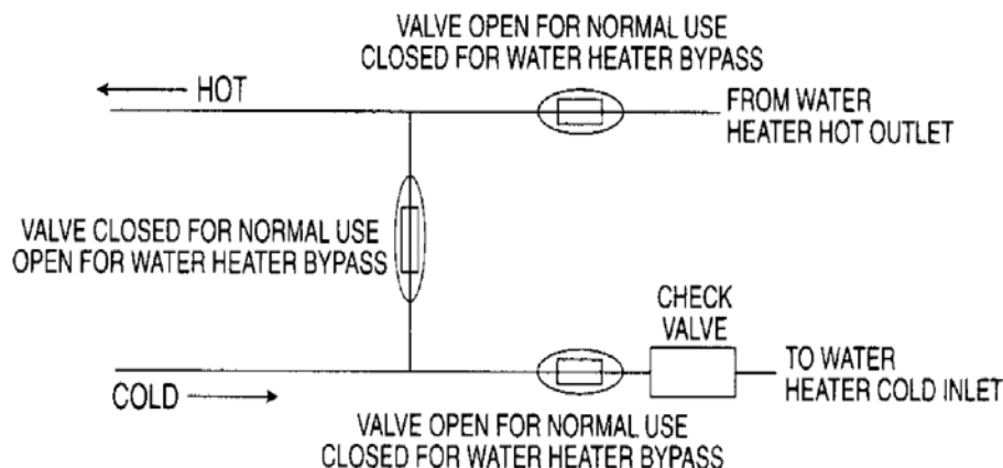
Schéma des vannes de dérivation du chauffe-eau
