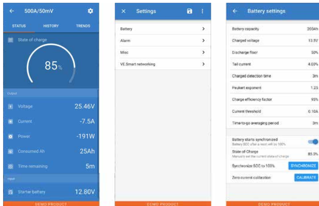
Les écrans de moniteur de batterie, surveillance et paramètres dans l'application VictronConnect.he battery monitor, monitoring, and setting screens in the VictronConnect app.
