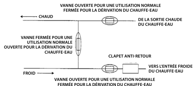
Schéma des vannes de dérivation du chauffe-eau
