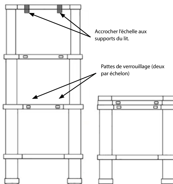
Échelle de couchette télescopique, montrée escamotée et prête à être utilisée.
