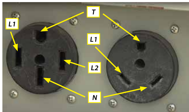
Prise de service électrique de 50 ampères, 240 volts
