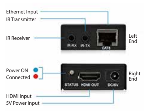
Ports d'entrée/sortie de récepteur typiques
