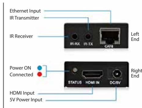
Ports d'entrée/sortie d'émission typiques
